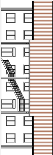
Prospetto SUD
