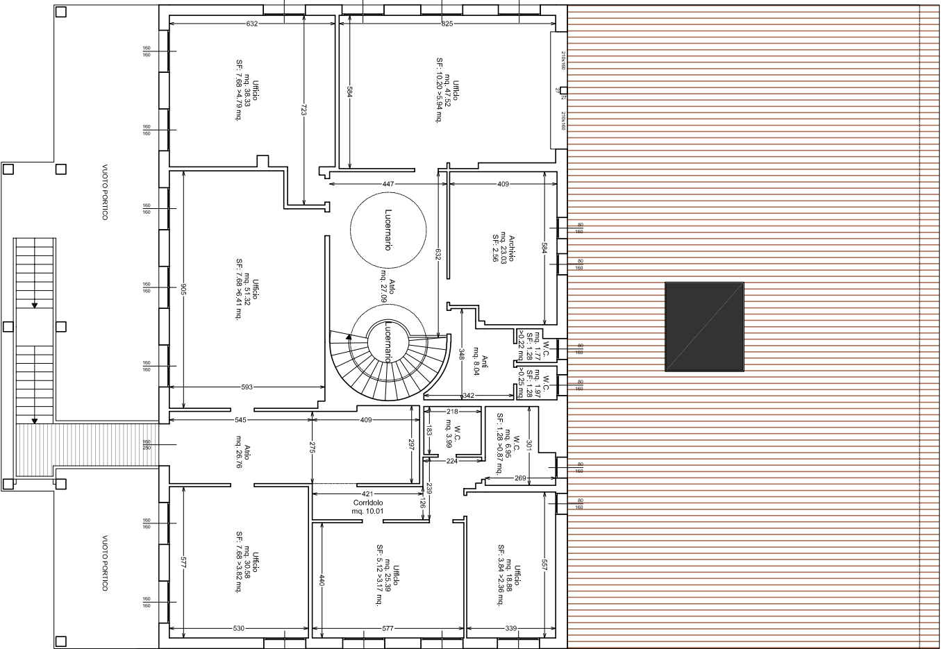
PIANTA PIANOPRIMO
