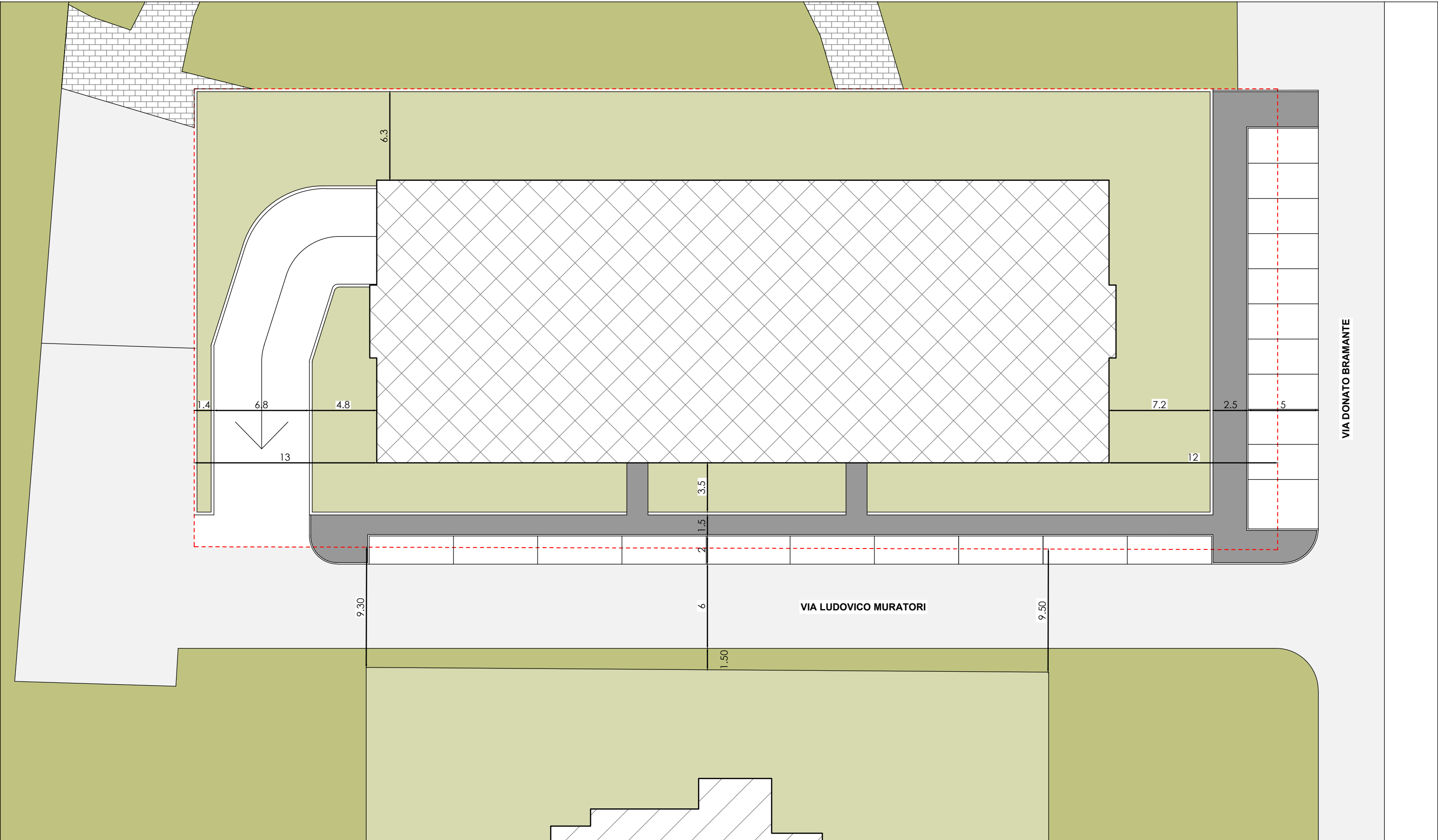
SISTEMAZIONE ESTERNA CONCESSIONATO (CON APPROVAZIONE PROPOSTA DI MODIFICA SEDIME FABBRICATO A PROTOCOLLO 27636 DEL 10 MAGGIO 2011) SCALA 1:250
