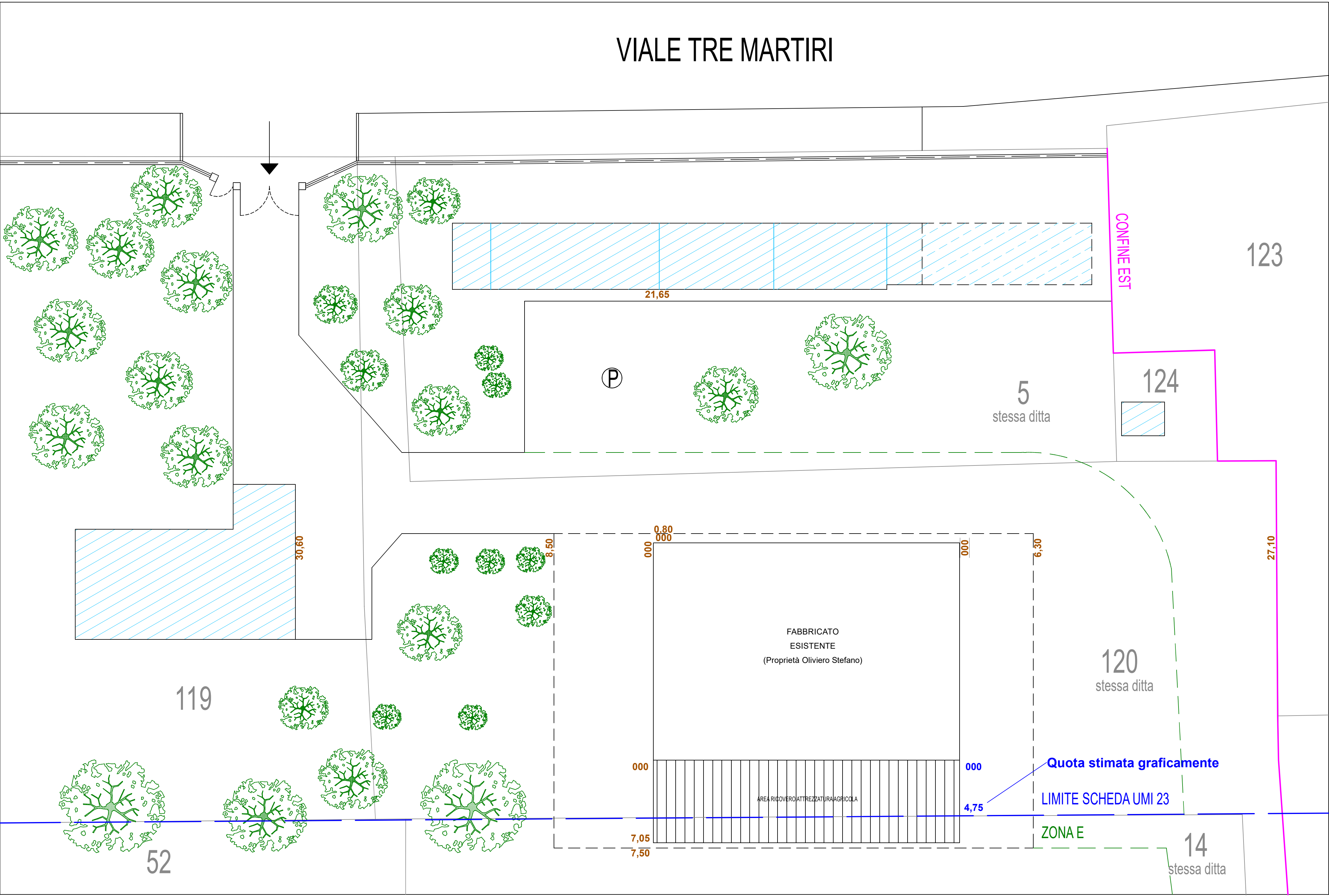
PLANIMETRIA SISTEMAZIONE ESTERNA sc. 1:200
