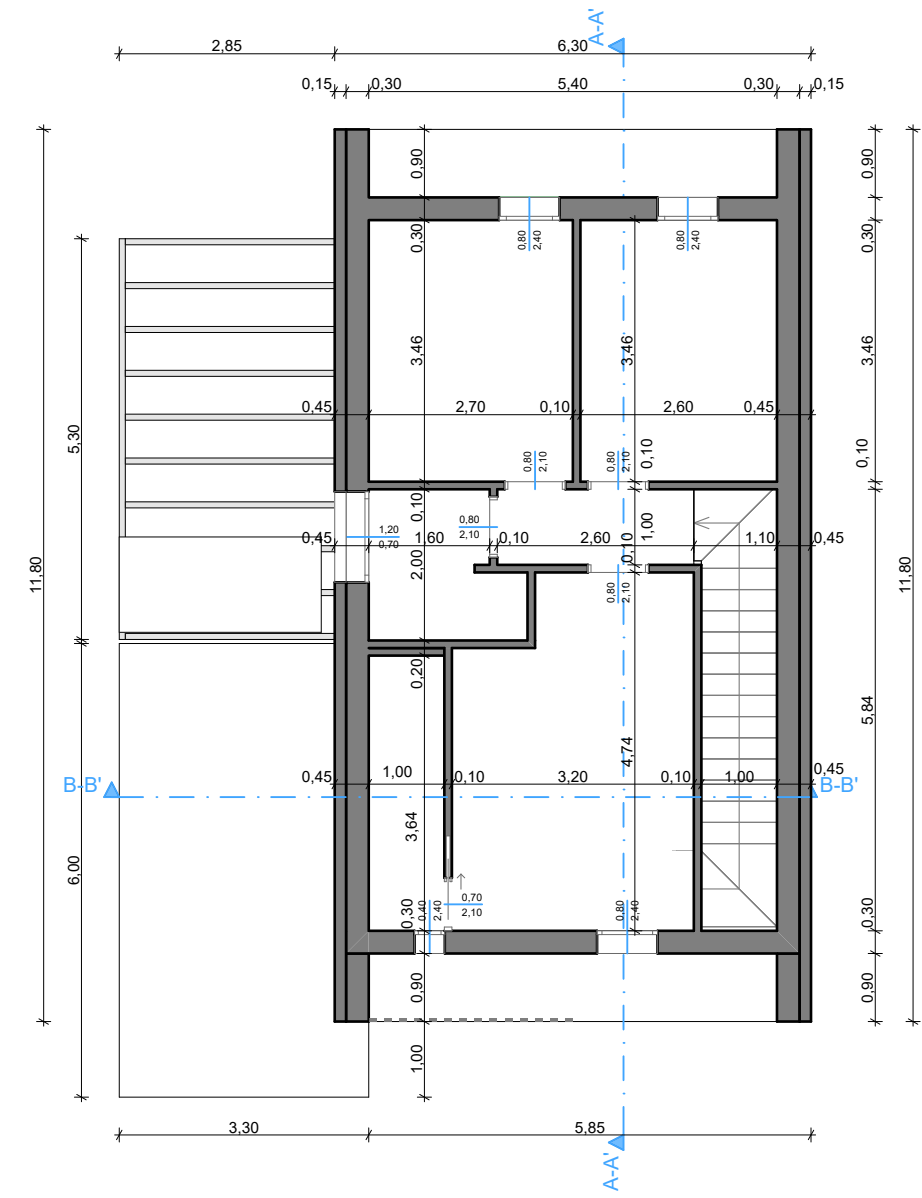
1. PIANO PRIMO 1:100
