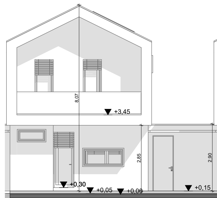
PROSPETTO NORD 1:100
