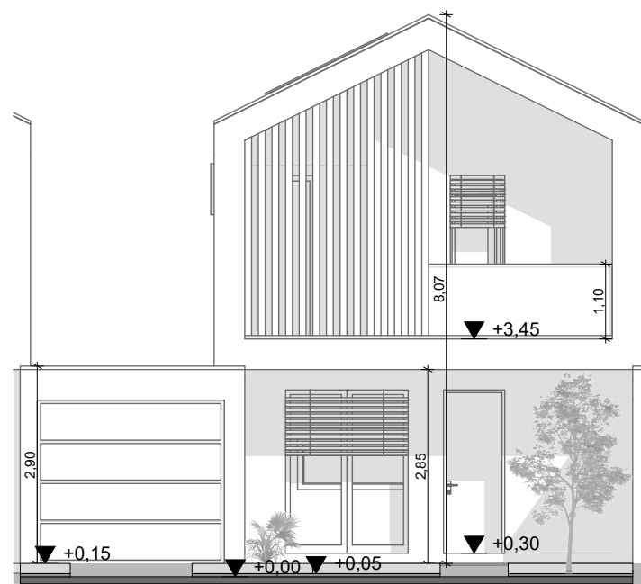
PROSPETTO SUD 1:100
