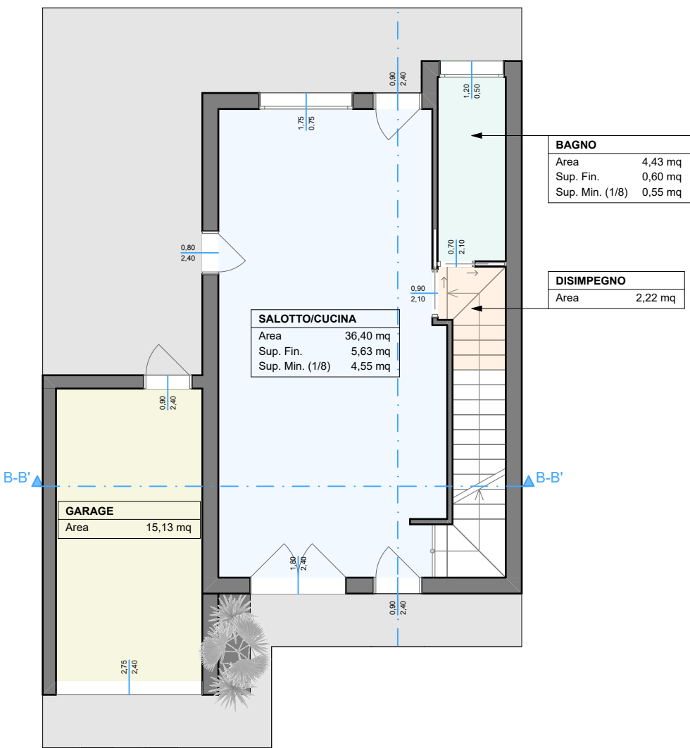
zone funzionali PIANO TERRA 1:100
