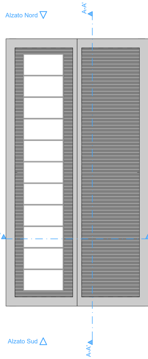
2. COPERTURA 1:100
