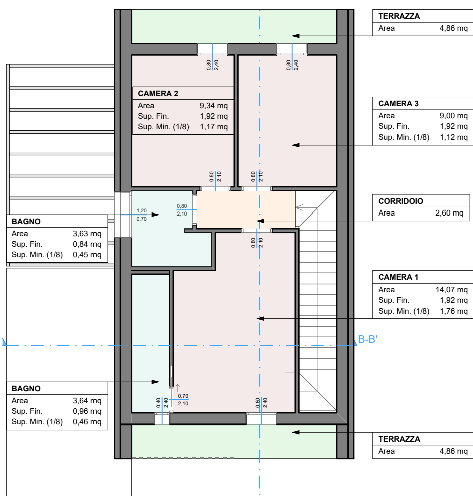
zone funzionali PIANO PRIMO 1:100
